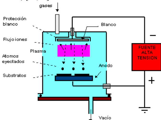
Figura2. Esquema experimental de deposición por Magnetron Sputtering. [9]
