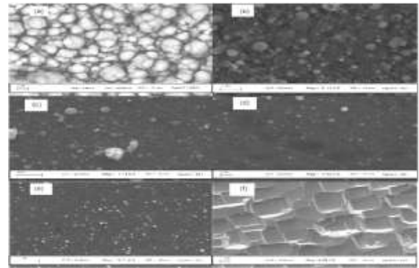
Figura 6. Imágenes SEM de películas delgadas de AlN depositadas por PLD a varias presiones: (a) 100 Torr; (b) 50 Torr; (c) 10 Torr; (d) 1 Torr; (e) 10^{-1} Torr; (f) 5 \times 10^{-2} Torr. [61]
