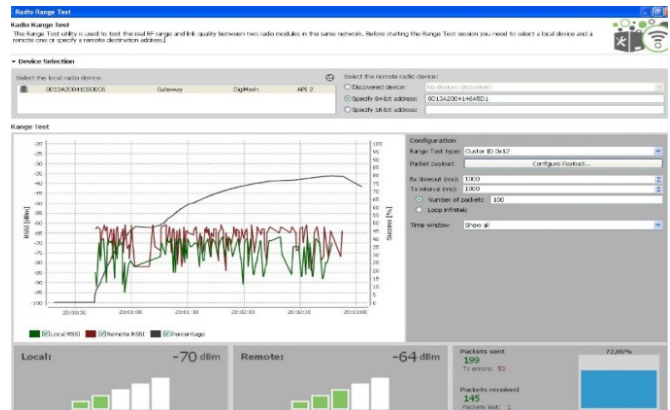
Fig. 14. Potencia Nodo 3 – Gateway.
