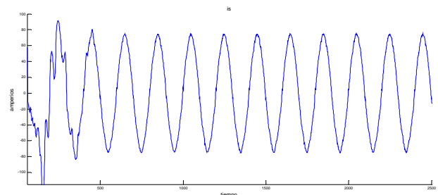
Figura 6. Corriente de la fuente de alimentación a 3300 Voltios con doble control
