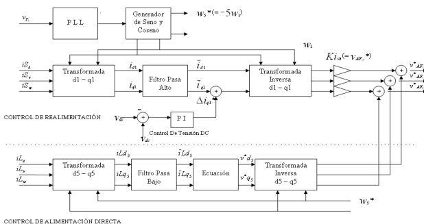
Figura 2. Esquema de control utilizado.
