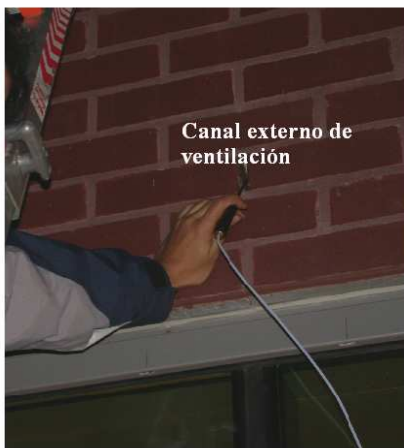
Figura 5. Posición del sensor para medición en el exterior del local.
