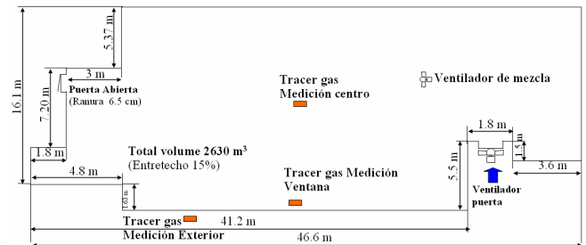
Figura 1. Dimensiones y posición de los sensores.
