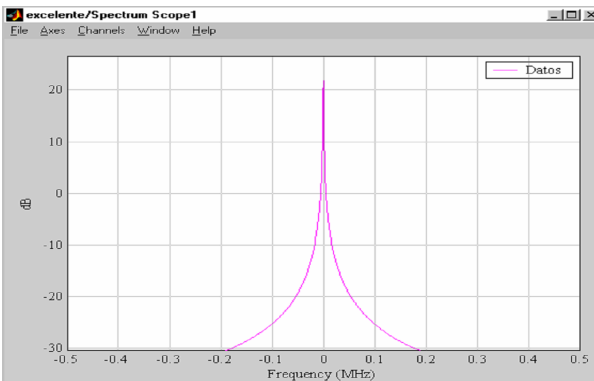
Figura 17. Espectro de la señal cuadrada utilizada como datos, mostrado por el Spectrum Scope del Simulink de MatLab®. Al igual que la imagen obtenida en el Fluke View (ver figura 12), se observa un espectro reducido de alta potencia.
