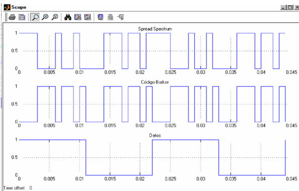
Figura 16. Resultado mostrado por el Scope del Simulink de MatLab®, de la señal en Spread Spectrum, el código Barker y la señal cuadrada utilizada como datos, respectivamente. Compárese con las imágenes 9, 10 y 11, obtenidas en el escopómetro.
