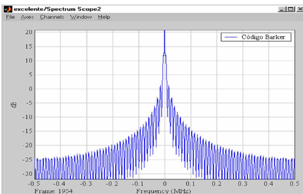
Figura 18. Espectro del código Barker generado, mostrado por el Spectrum Scope del Simulink de MatLab®. Al igual que la imagen obtenida en el software Fluke View (ver figura 13), se observa un espectro más amplio con la potencia distribuida en todos sus armónicos.
