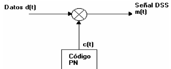
Figura 2. Transmisión de DSSS en banda base
