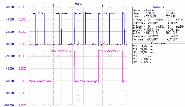
Figura 9. Imagen del código Barker (canal A en color azul) y la señal cuadrada utilizada como datos (canal B en color rosa). Obsérvese que todo el código Barker (10110111000) se repite durante cada bit de datos.
