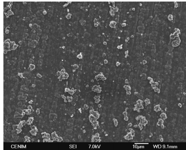
Figura 3a. Micrografía SEM de depósito de PPy con partículas de \text{Fe}_3\text{O}_4 incorporadas, sin presencia de \text{FeCl}_3 . Depósito obtenido galvanostáticamente a una corriente de 1\text{ mA} . Experimento E.
