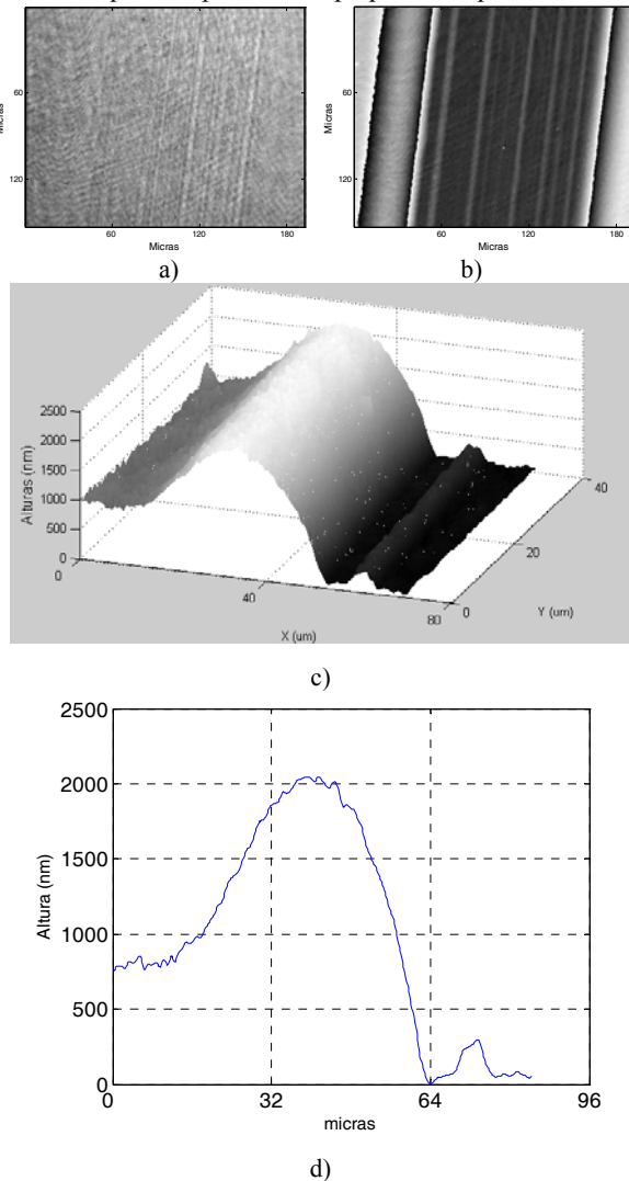
Figura 3. Aplicación de la técnica holográfica a la medida de espesores. a) Imagen de amplitud b) imagen de fase envuelta c) perfil de alturas 3-D d) perfil del escalón en una línea.
