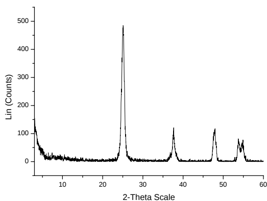
Figura 2. Espectro de Difracción de Rayos X del polvo de \text{TiO}_2 obtenido a partir de la solución sol-gel.
