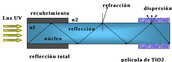
Figura 1. Diagrama de los procesos que ocurren en una fibra óptica con su recubrimiento original, sin recubrimiento y con \text{TiO}_2 soportado.
