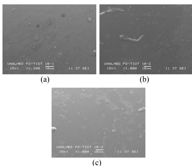
Figura 4. Imágenes SEM para las fibras soportadas por el método sol-gel: (a) 1 capa, (b) 2 capas y (c) 3 capas.
