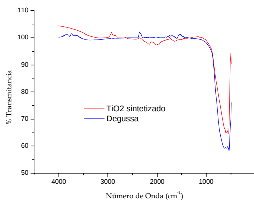
Figura 3. Espectro Infrarrojo del polvo de \text{TiO}_2 obtenido a partir de la solución sol-gel.
