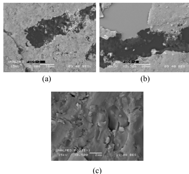
Figura 5. Imágenes SEM para las fibras soportadas por inmersión a partir de suspensiones de \text{TiO}_2 comercial, Degussa P-25: (a) 5 % con 3 capas, (b) 8 % con 2 capas y (c) 11 % con 1 capa.
