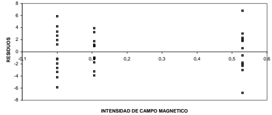
Figura 7. Gráfico de Residuos contra Intensidad de Campo Magnético
