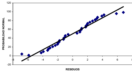
Figura 4. Grafica de Probabilidad normal de los residuos
