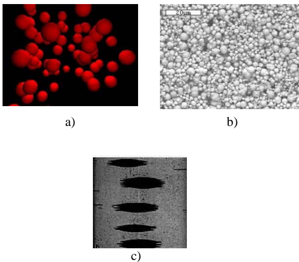
Figura 1. Micrografías del comportamiento de un fluido MR ante un campo magnético.
