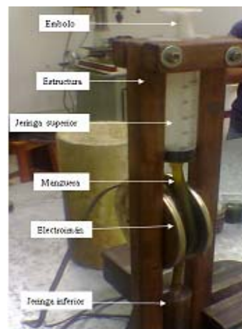
Figura 3. Dispositivo para medición de caudal
