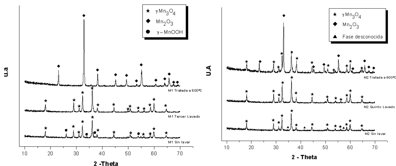
Figura 4: Difractograma de rayos X correspondientes a muestras sólidas M1 (Lavadas con agua + 0.05M de dietilamina) (a) y M2 (Lavada con etanol + 0.05M de dietilamina) (b), tanto del precipitado como de los sólidos obtenidos de los lavados y tratados térmicamente a 600 °C.
