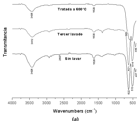
Figura 3: Espectros FTIR correspondientes a las muestras sólidas M1 (a) y M2 (b), tanto del precipitado como de la muestra lavada varias veces, como de la tratada térmicamente a 600 °C
