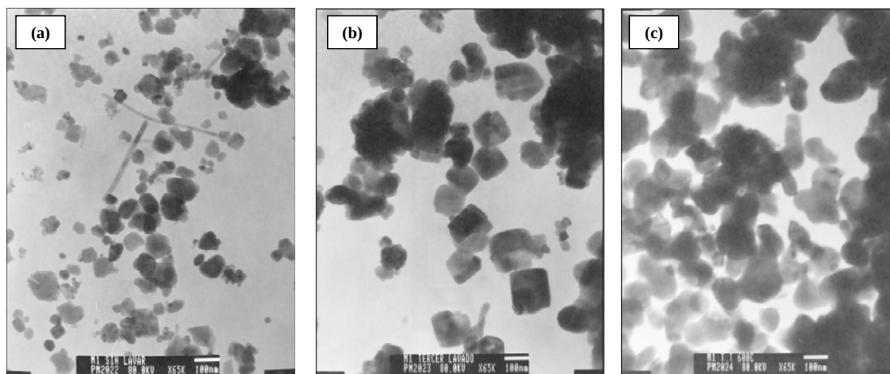
Figura 5: Fotografías obtenidas con MET para las muestras sólidas M1 precipitada con \text{NH}_4\text{OH} y secada sobre una plancha calefactora a 60°C. (a) Lavada tres veces con agua + 0.05M de dietilamina (b), tratada térmicamente a 600 °C durante 24 horas (C).
