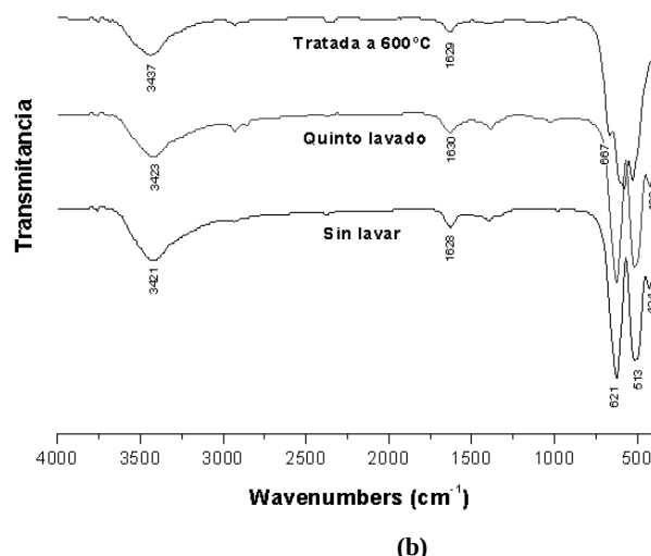
Figura 3: Espectros FTIR correspondientes a las muestras sólidas M1 (a) y M2 (b), tanto del precipitado como de la muestra lavada varias veces, como de la tratada térmicamente a 600 °C
