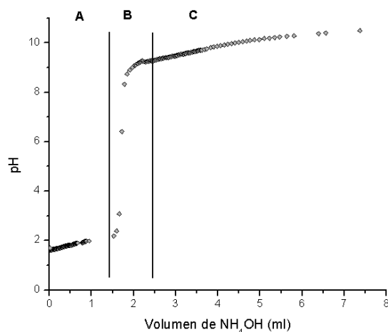
Figura 1: Curva de valoración potenciométrica obtenida para la solución 0.1M de MnCl_2 + 4H_2O .
