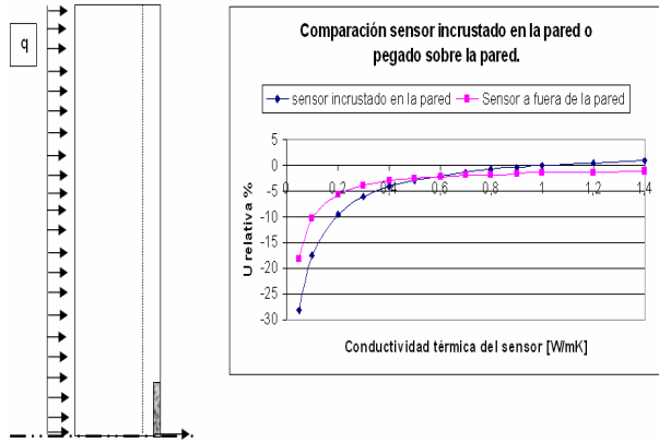
Figura 9. Sensor incrustado
