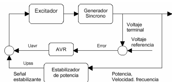
Figura 1. Control de la excitación en una máquina síncrona mediante operación conjunta de AVR y estabilizador
