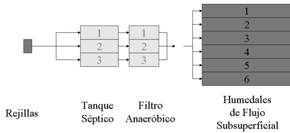
Figura 1. Componentes de la PTAR.
