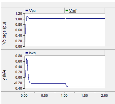
Figura 6. Punto de equilibrio al conectar el SVC
